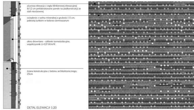
DETAL ELEVACJI 1:20
