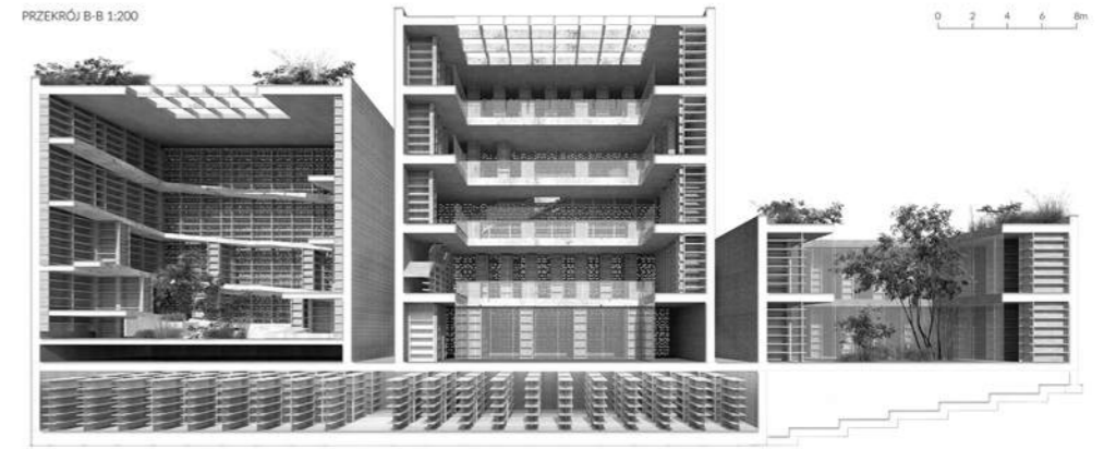
PRZEKROJ B-B 1:200
