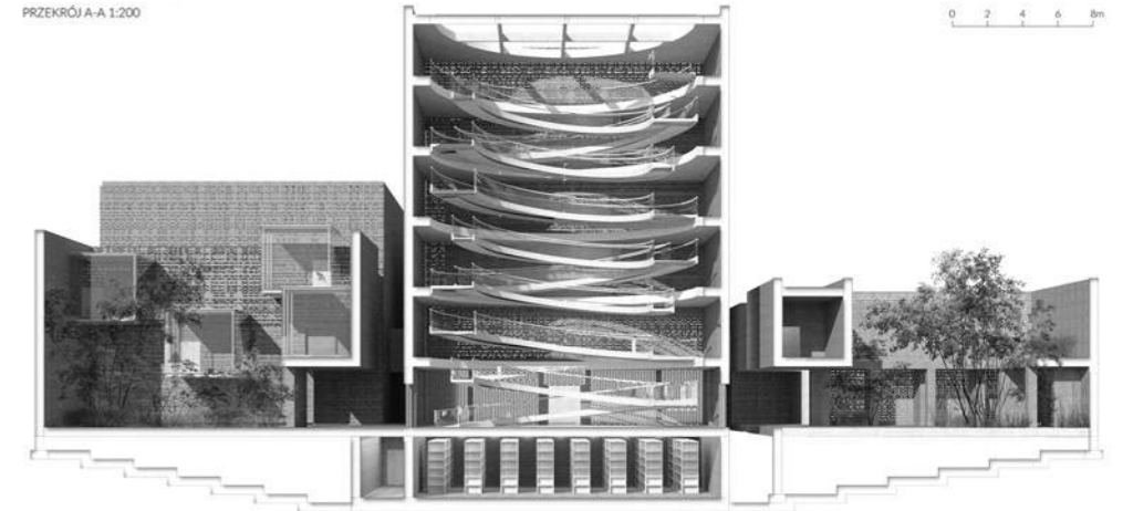
PRZEKROJ A-A 1:200
