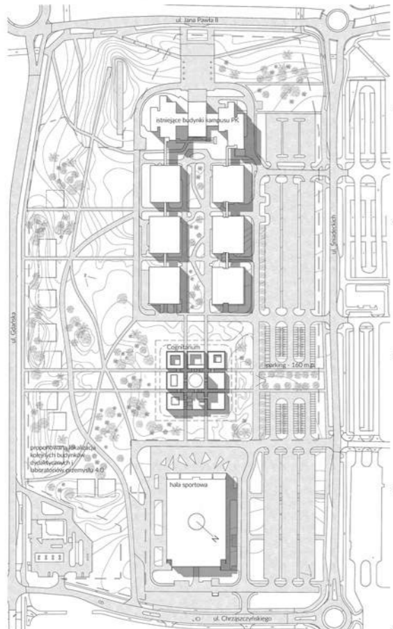
PLAN SYTUACYJNY 1:2000
